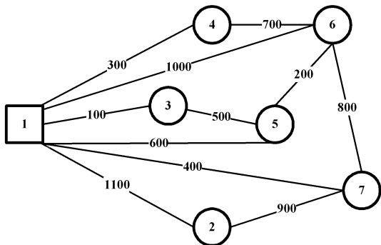
题 35 图:某住宅区安装供水管道线路图
