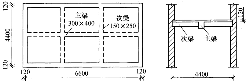
题 41 图 麻刀石灰浆面层井字梁天棚
