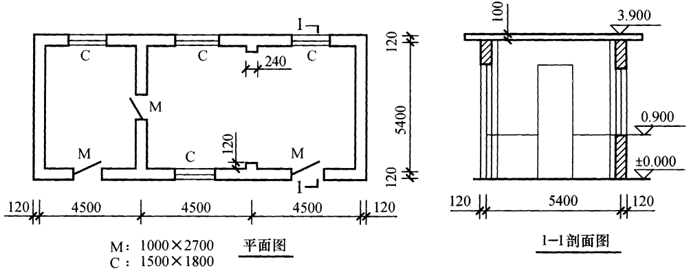
题 40 图 办公用房抹灰
