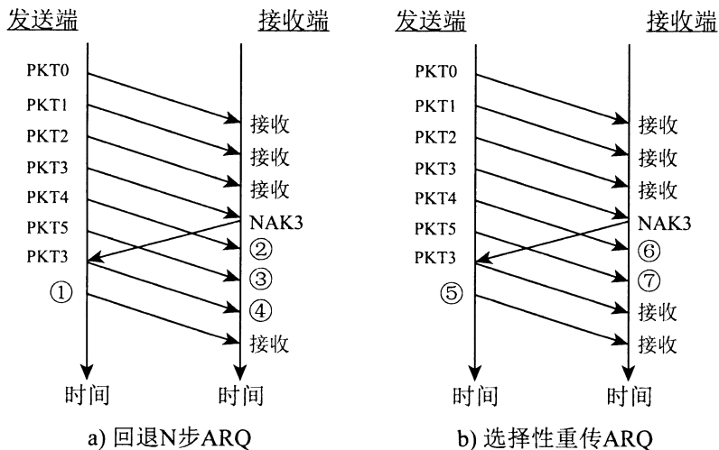
题 27 图 ARQ 工作原理示意图
